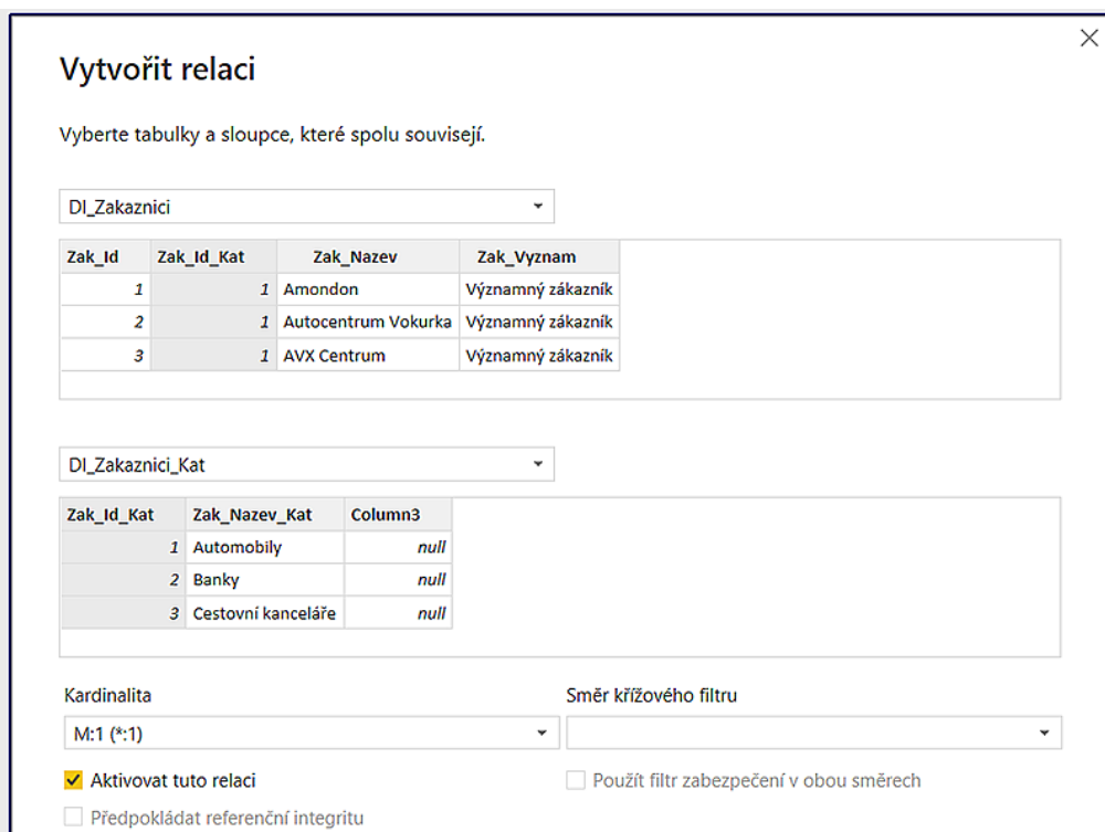
Obrázek 4-9: Vytvoření vztahu mezi entitami
