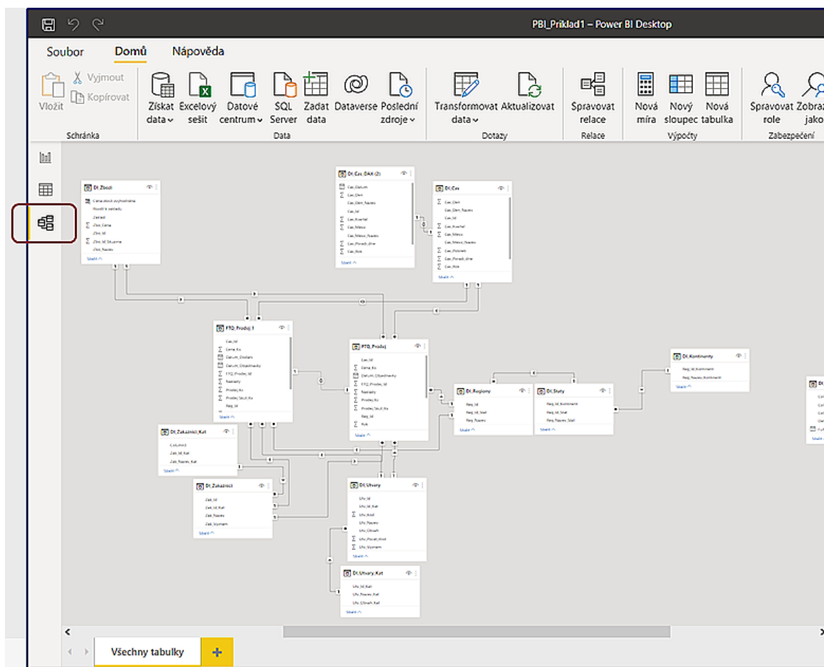
Obrázek 4-7: Automaticky vytvořený datový model po načtení datových zdrojů do Power BI
