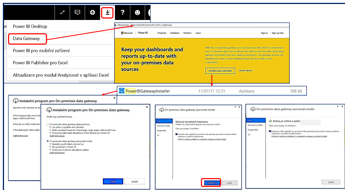
Obrázek 6-1: Instalace a zpřístupnění DataGateway
