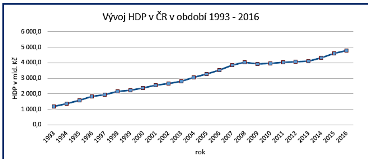
Obrázek 8-21: Spojnicový diagram
