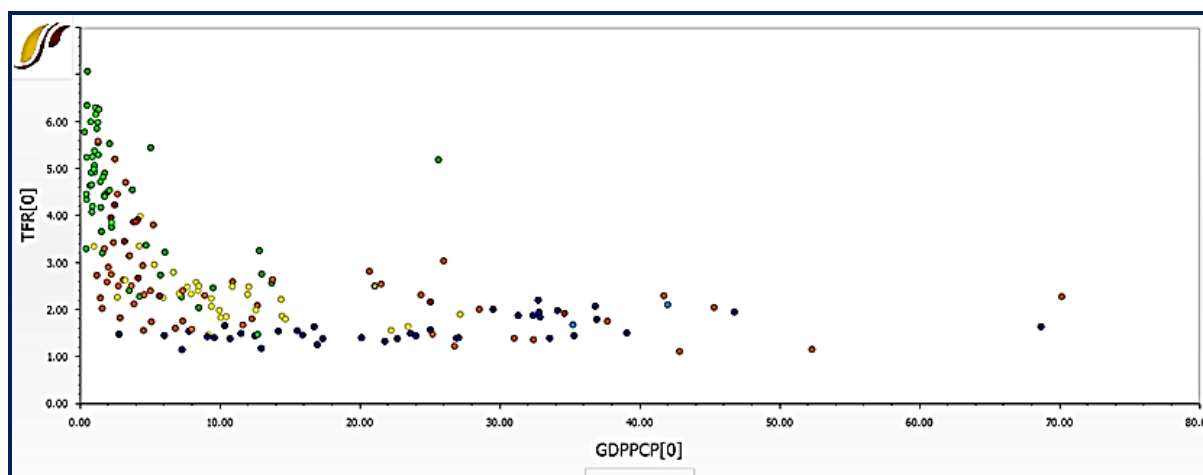
Obrázek 8-26: Bodový graf
