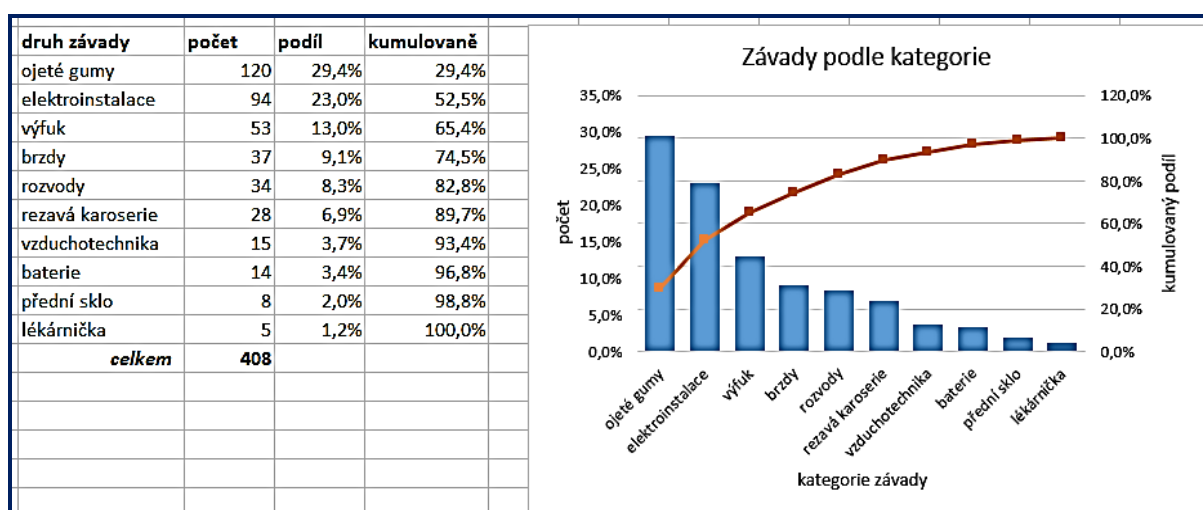
Obrázek 8-23: Paretův diagram
