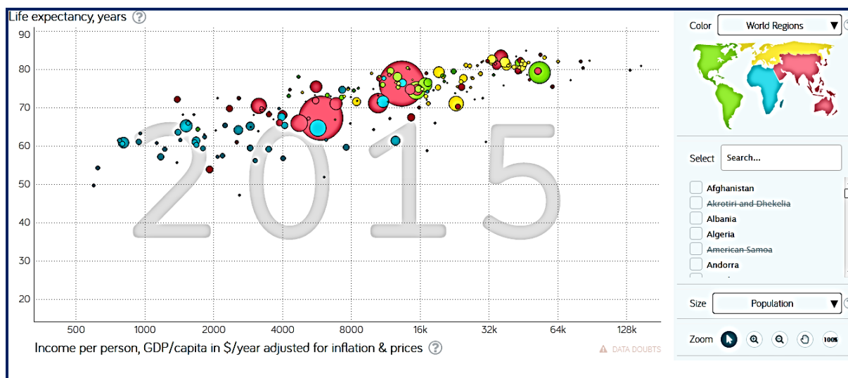
Obrázek 8-29: Bublinový graf
