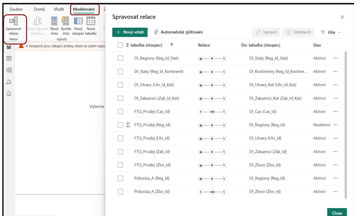
Obrázek 4-9: Správa relací
