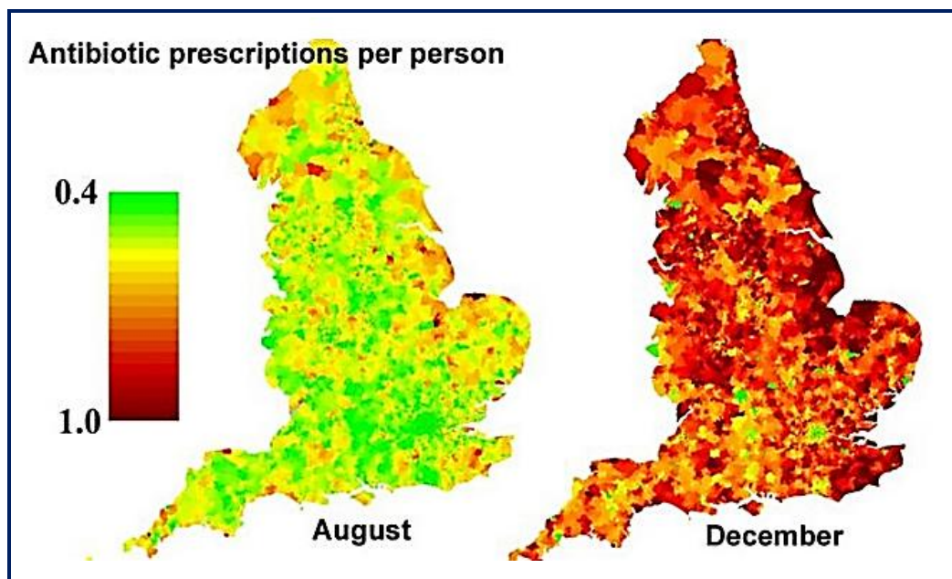
Obrázek 8-28: Teplotní mapa
