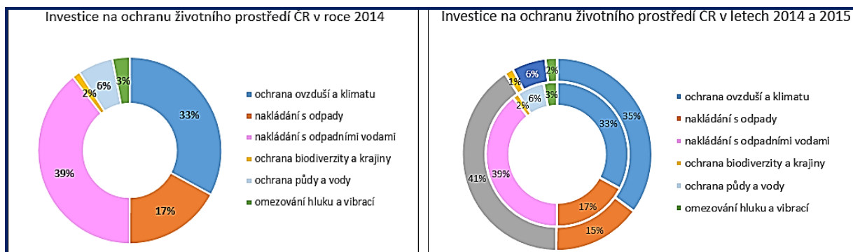
Obrázek 8-20: Prstencový graf
