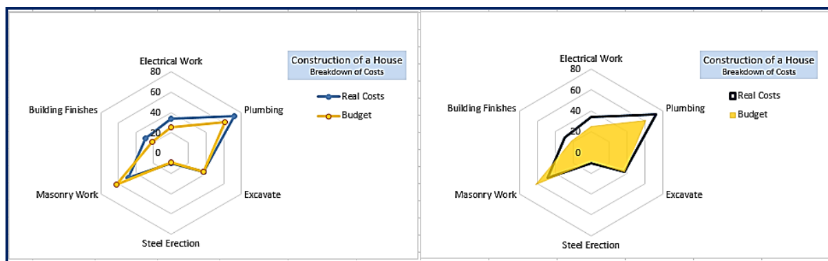
Obrázek 8-25: Paprskový graf
