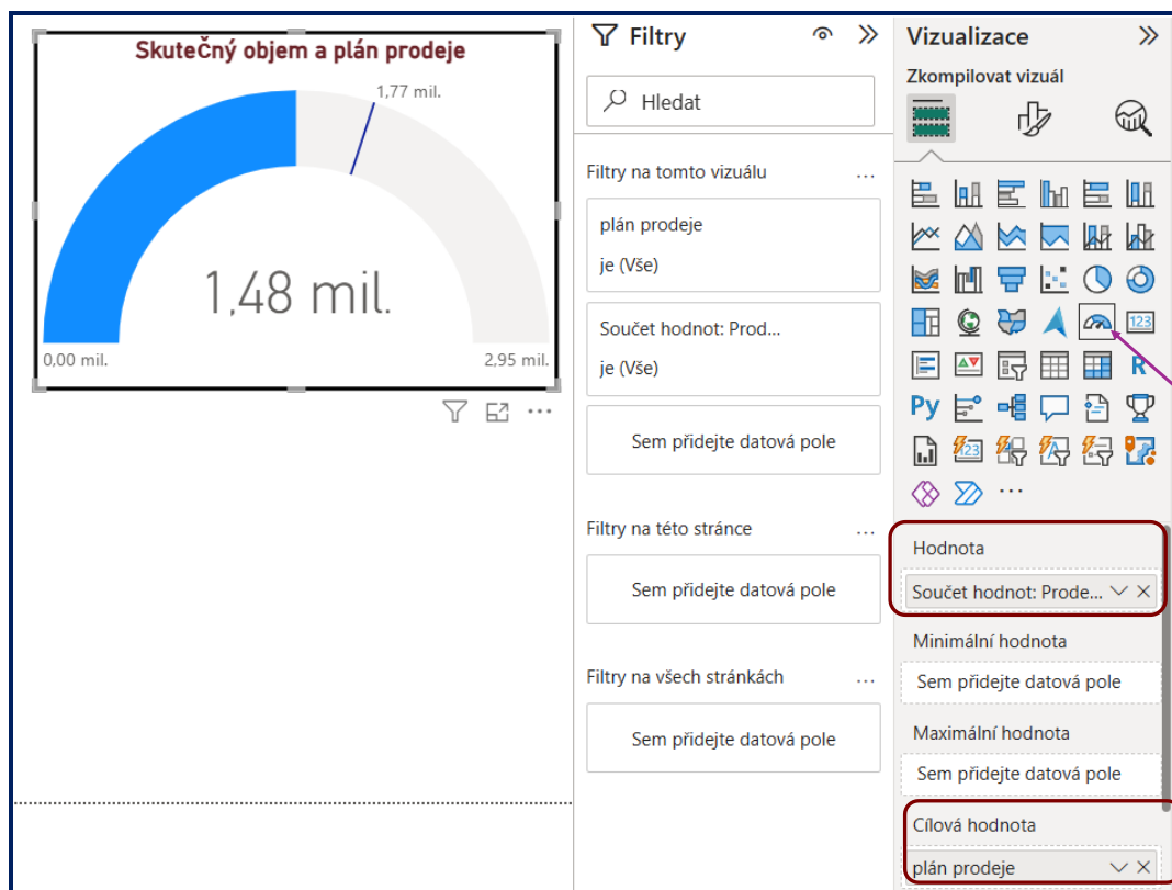
Obrázek 5-7: Měřidlo (Gauge)
