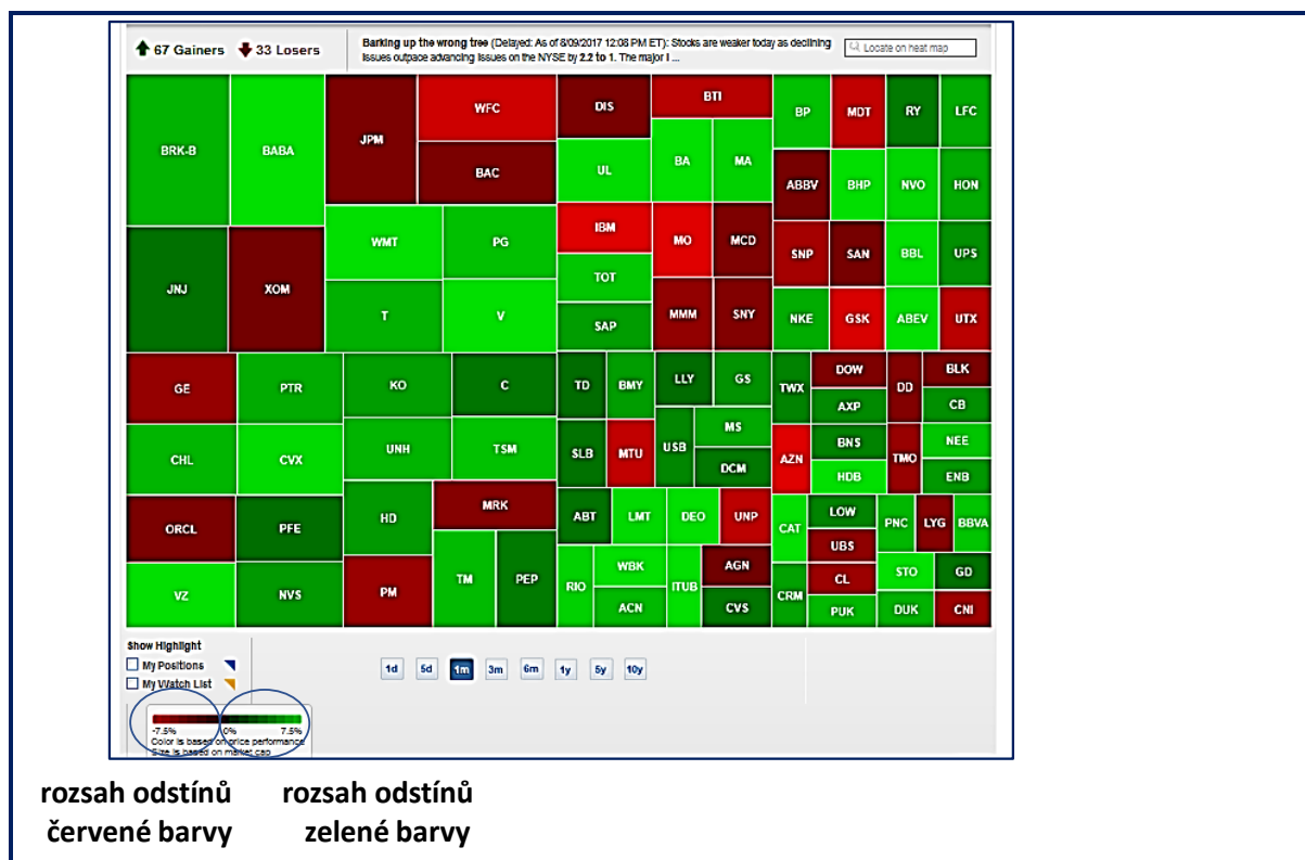
Obrázek 8-31: Stromová mapa
