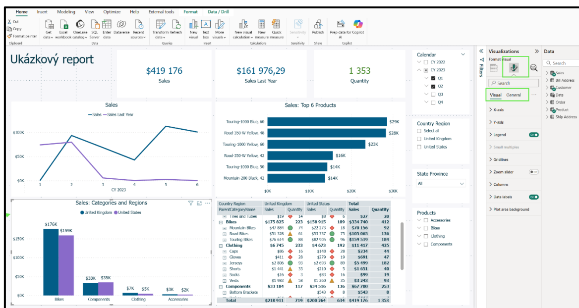
Obrázek 5-2: Formátování vizuálů
