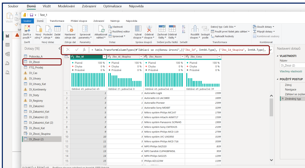
Obrázek 4-5: Power Query editor Power BI Desktop
